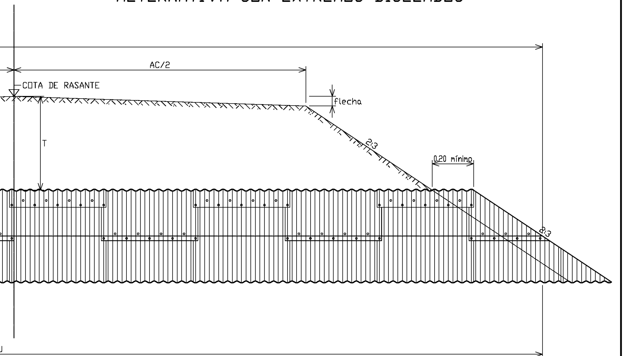
ALTERNATIVA CON EXTREMOS BISELADOS
