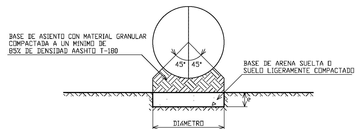
3 - FUNDACIÓN SOBRE TERRENO ROCOSO
