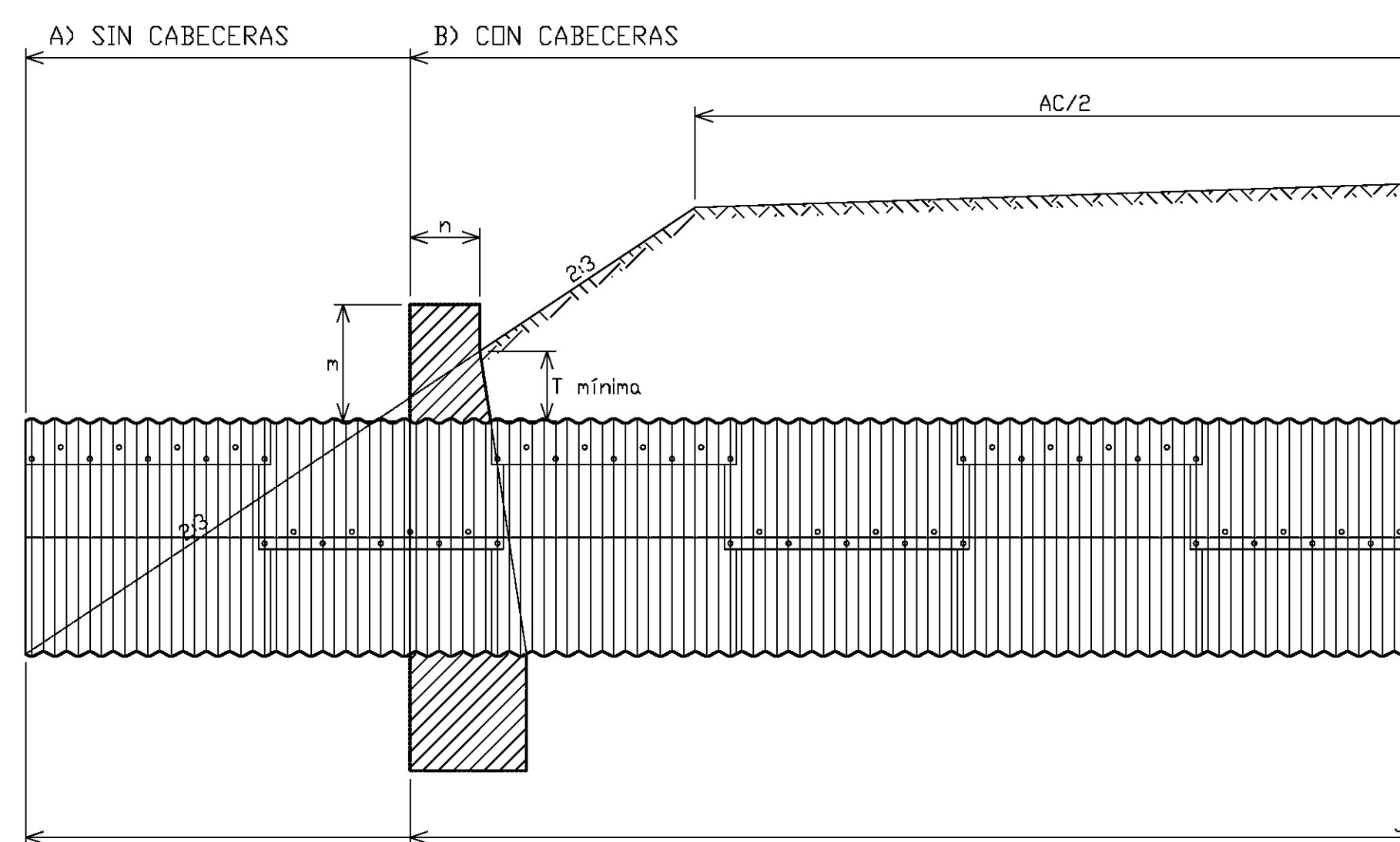
ALTERNATIVAS CON EXTREMOS RECTOS
