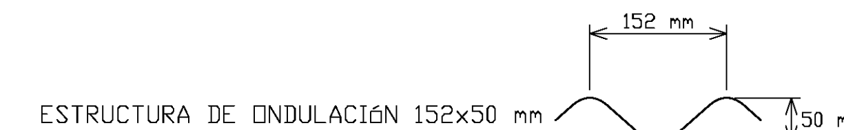
ESTRUCTURA DE ONDULACIÓN 152x50 mm
