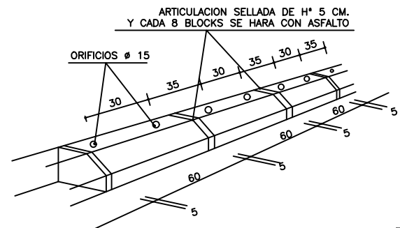
"CORDON TIPO H"
