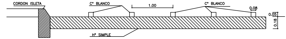
CORTE A-A
