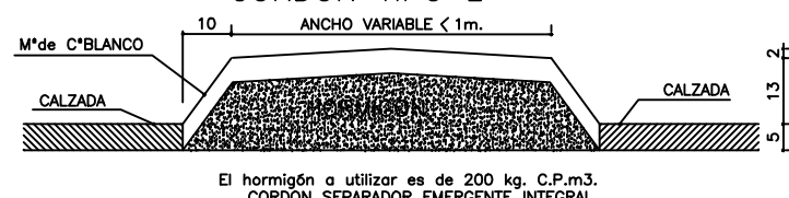
"CORDON TIPO L"
