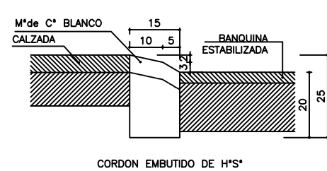
CORDON EMBUTIDO DE H°S°
