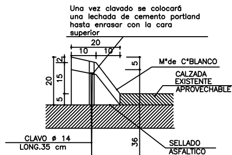
CORDON PREMOLDEADO PARA APLICAR SOBRE PAVIMENTO EXISTENTE
